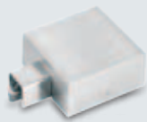
Endeinspeisung L. 11,5 cm, B. 8,5 cm, H. 4 cm, max. 2x1.800 W 8243564 € 89,95
